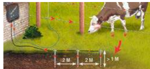
Toma de tierra pequeño modelo ref. 667.602
