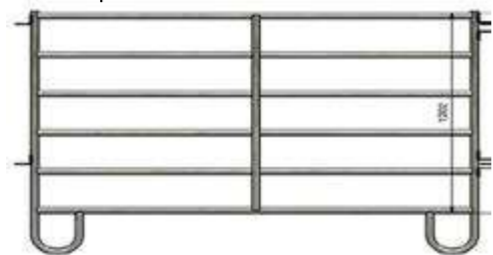
Panel Contencion tubo 34mm Galva 2.0 y 3.0m Altura 1.60m. Union con 1 varilla incluida.
