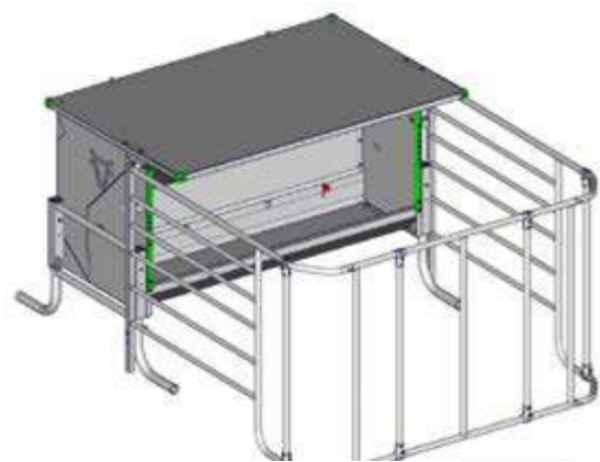
Tolva Terneros Selectiva. con o sin parque. Capacidad y medidas incluyendo parque 2.20x3.15m 950lt y 3.0m 1350lt.
