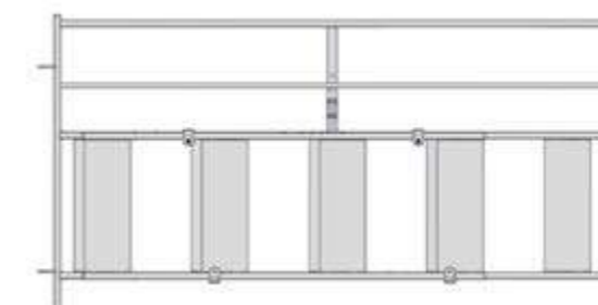
Valla telera con paso de corderos regulable 2.0m
